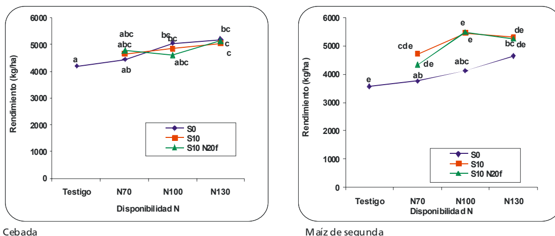
Figura 10: Rendimientos de la secuencia cebada-maíz, resultado de diferentes disponibilidades de nitrógeno inicial (suelo + fertilizante), azufre (como fertilizante) y nitrógeno foliar. Los tratamientos fueron aplicados en cebada. El maíz fue refertilizado de manera uniforme con 19 kg P y 64 kgN ha -1 . La Trinidad, General Arenales, campaña 2006/07. Tomado de Ferraris et al, 2007.
