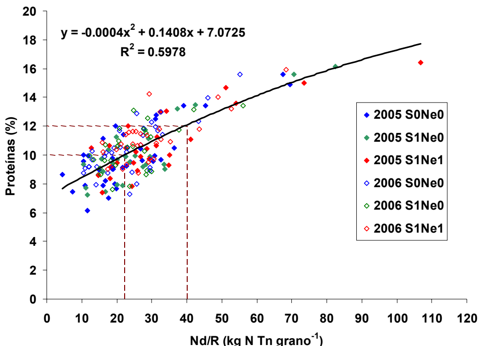
Figura 4: Relación entre el contenido proteico de los granos y el cociente entre la disponibilidad inicial de N en el suelo más el aportado por el fertilizante y el rendimiento obtenido (Nd/R). Se indica la ecuación ajustada ( n = 183 ). Cada punto indica la media de las 3 o 4 (de acuerdo al experimento) parcelas.
