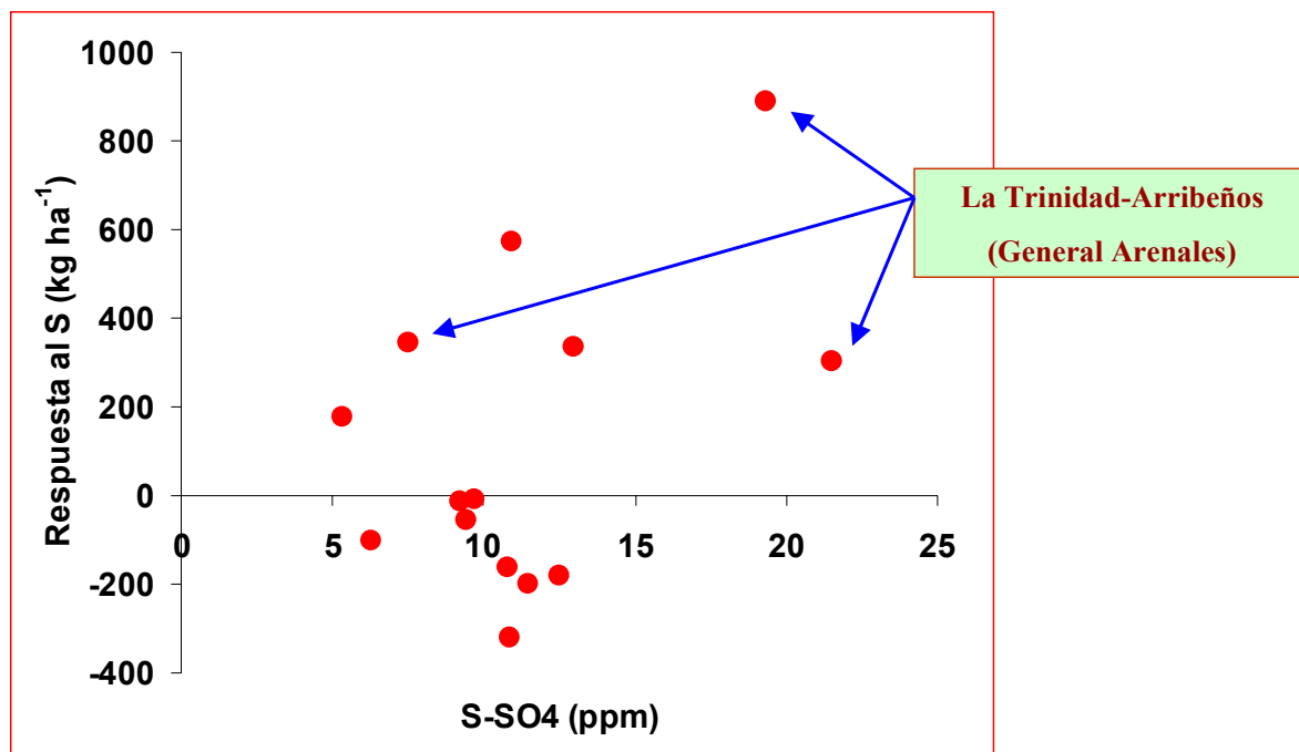
Figura 7: Respuesta a la fertilización azufrada en función de la concentración de S-SO_4^- presente en la capa de 0 a 20 cm del suelo durante la siembra. Las flechas señalan sitios de alto rendimiento localizados en el partido de General Arenales, con diferencias positivas por agregado de azufre. Tomado de Gutiérrez Boem et al., 2008.
