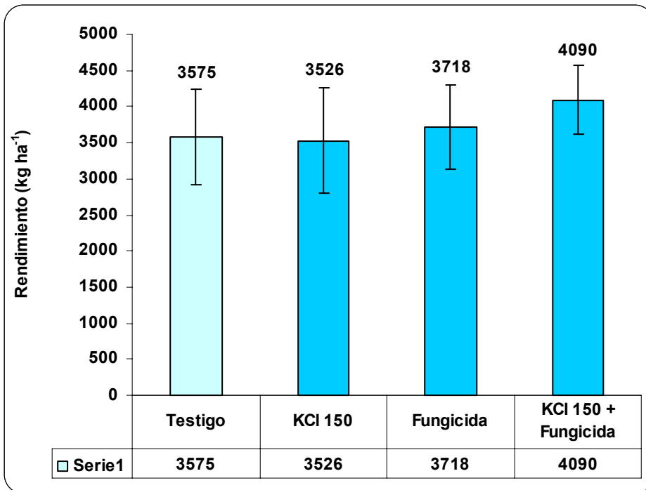
Figura 8: Rendimientos como resultado de la aplicación de cloruro de potasio a la siembra en combinación con fungicidas en cebada, en la localidad de La Trinidad (General Arenales). Ferraris & Couretot, inédito.
